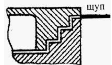
ступінчасте з'єднання
