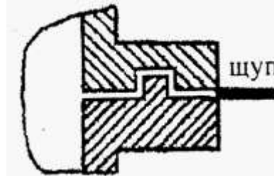
лабіринтне з'єднання
