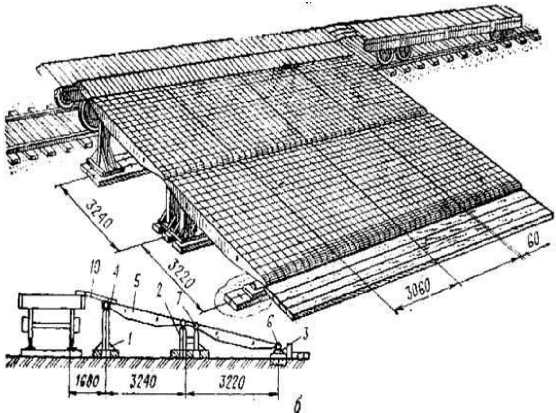
Мал. 2. Збірно-розбірна металева апарель а - торцева апарель; б - бокова апарель із чотирьох секцій
