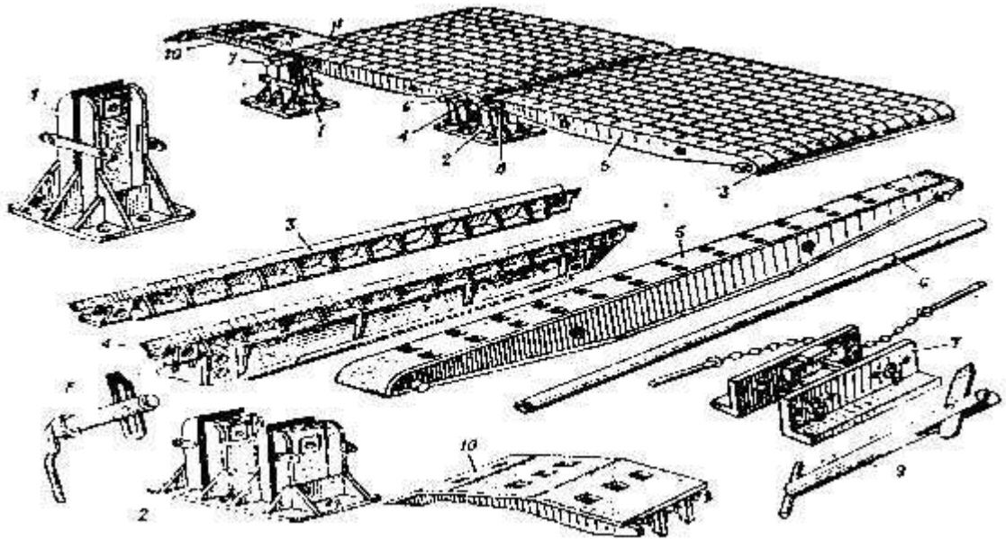
Мал. 1. Елементи збірно-розбірної металевої апарелі:
